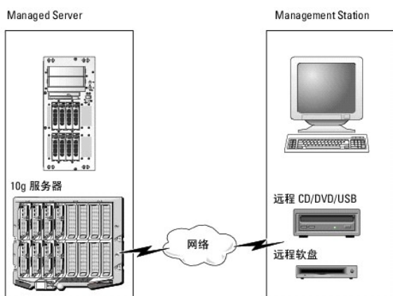
图 8-1. 虚拟介质的整体结构
